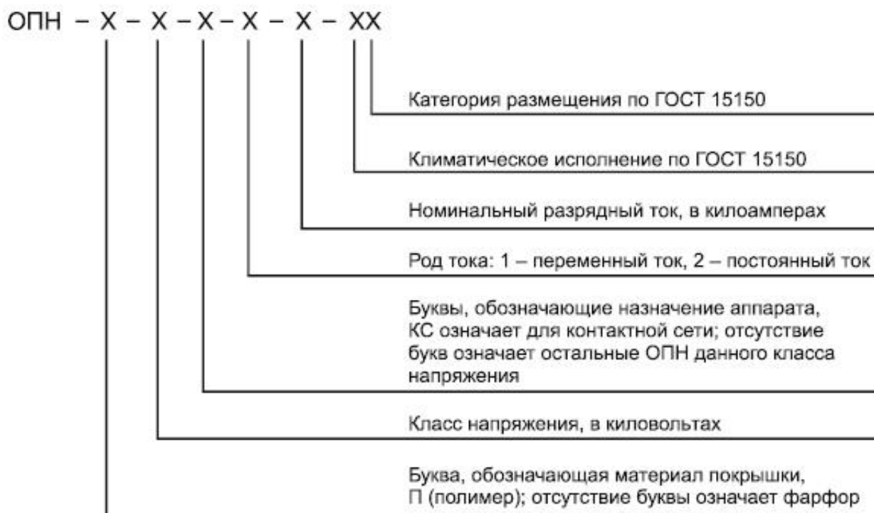
Рисунок 1 - Рекомендуемая структура условного обозначения ОПН
