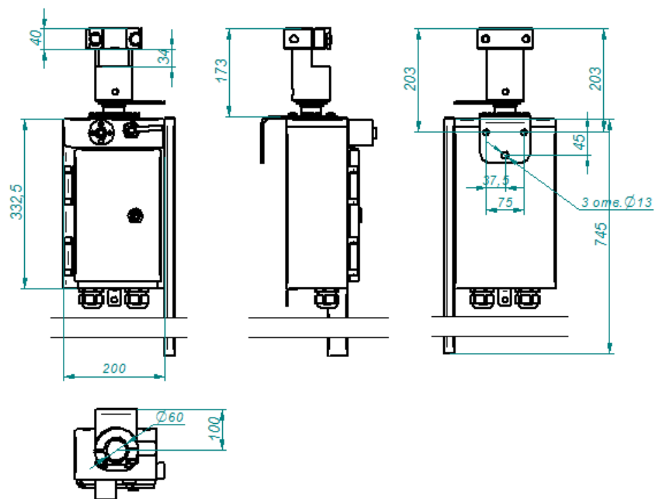
1. КОЛОДКА
