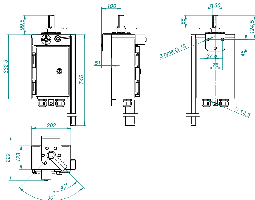
4. ЧЕТЫРЕХГРАННЫЙ ВАЛ только для ПРГ-5 серии
