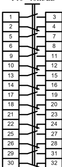
Рис.1. Электрическая схема.
