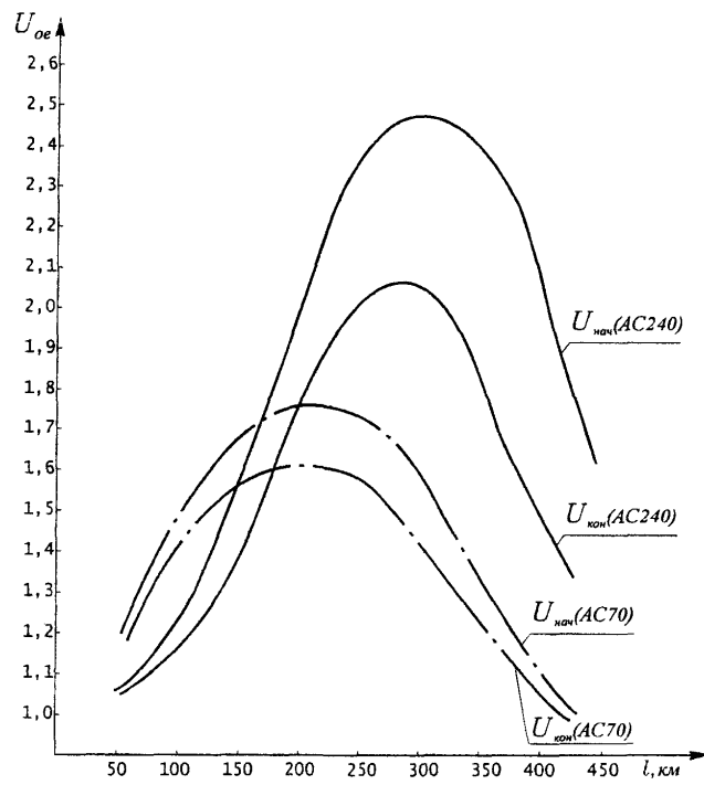
Рис. 8. Максимальные величины установившихся перенапряжений в полублочной схеме электропередачи 110 кВ при включении 2-х фаз ВЛ.
