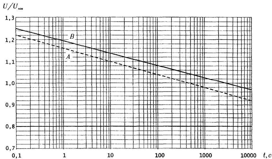
Рис. 1. Зависимость относительных величин временных перенапряжений U_n промышленной частоты, которые должны выдерживать ОПН EXLIM R, от их длительности.
