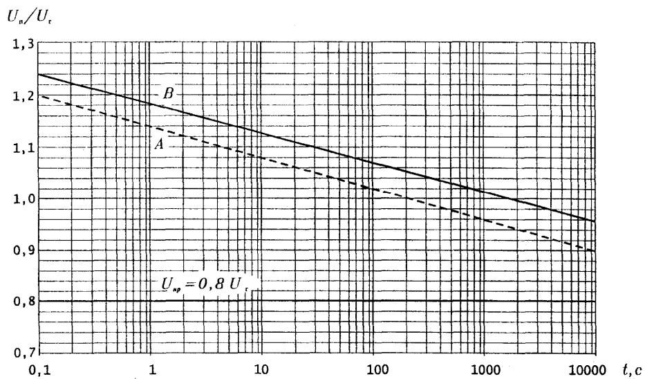
Рис. 3. Зависимость относительных величин временных перенапряжений U_n промышленной частоты, которые должны выдерживать ОПН EXLIM P, от их длительности.
