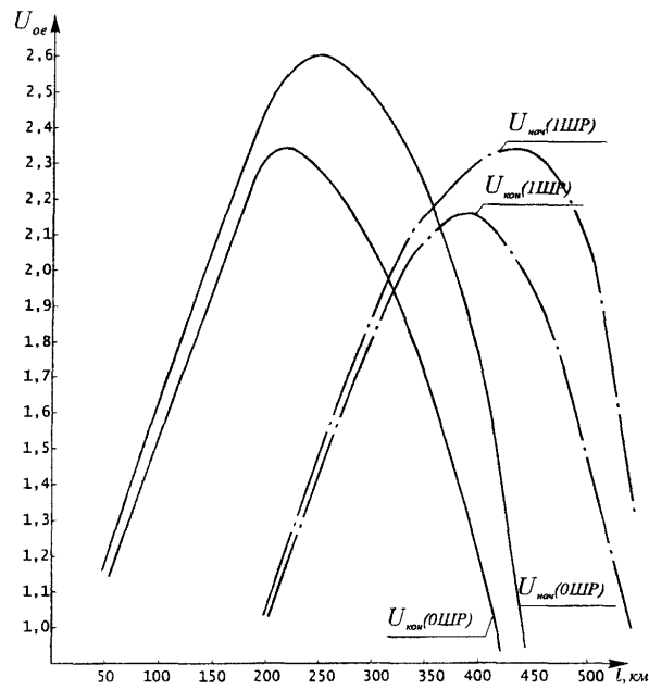
Рис. 10. Максимальные величины установившихся перенапряжений в полублочной схеме электропередачи 500 кВ при включении 2-х фаз ВЛ.
