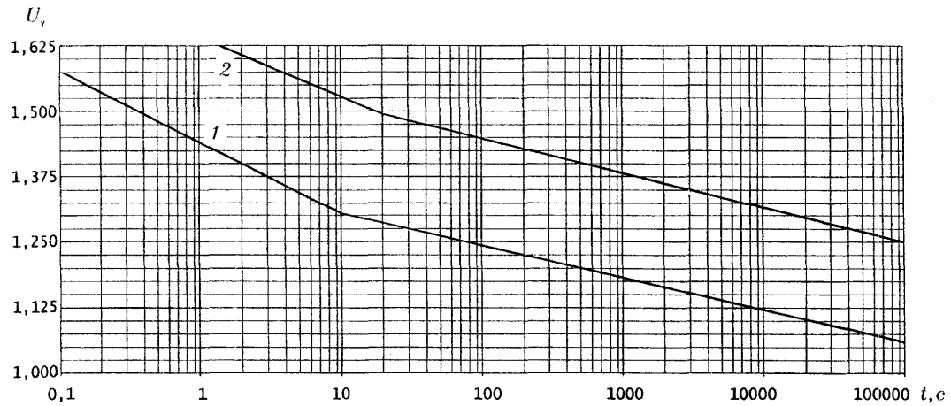
Рис. 5. Зависимость "допустимое напряжение - время" для случая без предварительного погружения импульсом энергии для ОПН, выпускаемых АООТ "КФЗ" по ТУ №: 1) 3414-019-04682628-97, 2) 3114-011-04682628-96.
