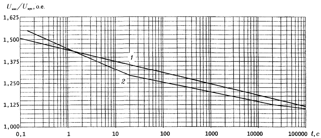
Рис. 6. Зависимость "допустимое напряжение - время" для случая: 1) предварительного нагрева и нагружения импульсом 2,5 кДж/кВ U_n для ОПН 110-220 кВ, выпускаемых ЗАО "Феникс-88" по ТУ 3414-007-06968694-97, 2) предварительного нагрева и нагружения импульсом 7,0 кДж/кВ U_n для ОПН 500 кВ, выпускаемых ЗАО "Феникс-88" по ТУ 3414-013-06968694-99.
