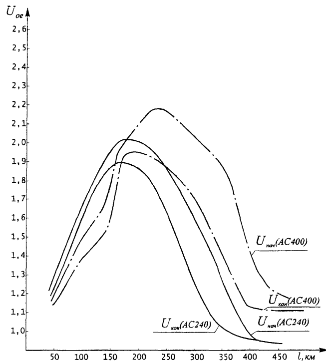
Рис. 9. Максимальные величины установившихся перенапряжений в полублочной схеме электропередачи 220 кВ при включении 2-х фаз ВЛ.
