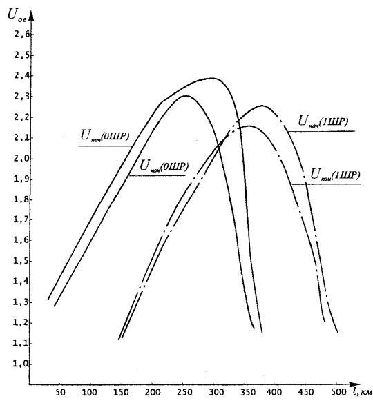
Рис. 11. Максимальные величины установившихся перенапряжений в полублочной схеме электропередачи 750 кВ при включении 2-х фаз ВЛ.
