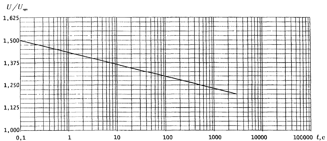
Рис. 7. Зависимость "допустимое напряжение - время" для случая предварительного нагружения импульсом 2,25 кДж/кВ U_{нрo} для ОПН, выпускаемых ООО "Таврида-Электрик" по
